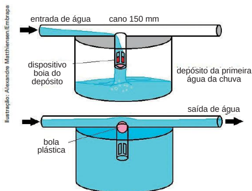
FIGURA 4 - ESQUEMÁTICO DE EXEMPLO DE DEPÓSITO PARA PRIMEIRA ÁGUA DA CHUVA, COM DISPOSITIVO BOIA. Fonte: EMBRAPA.
